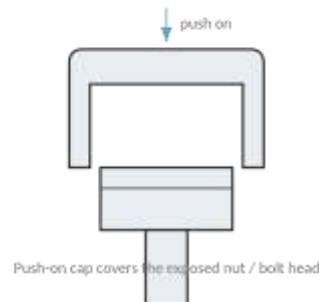
SECTION (PUSH-ON)
